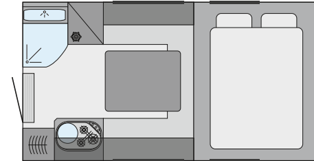
Inneneinrichtung TRAIL/BOX 240
