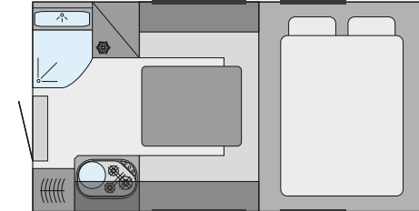
Inneneinrichtung TRAIL/BOX 220
