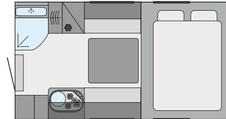
Inneneinrichtung TRAIL/BOX 280
